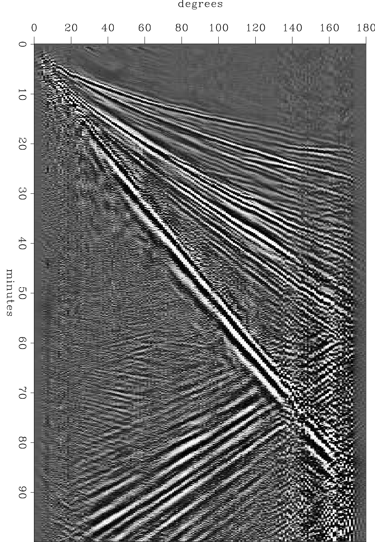
epsilon_is_2
