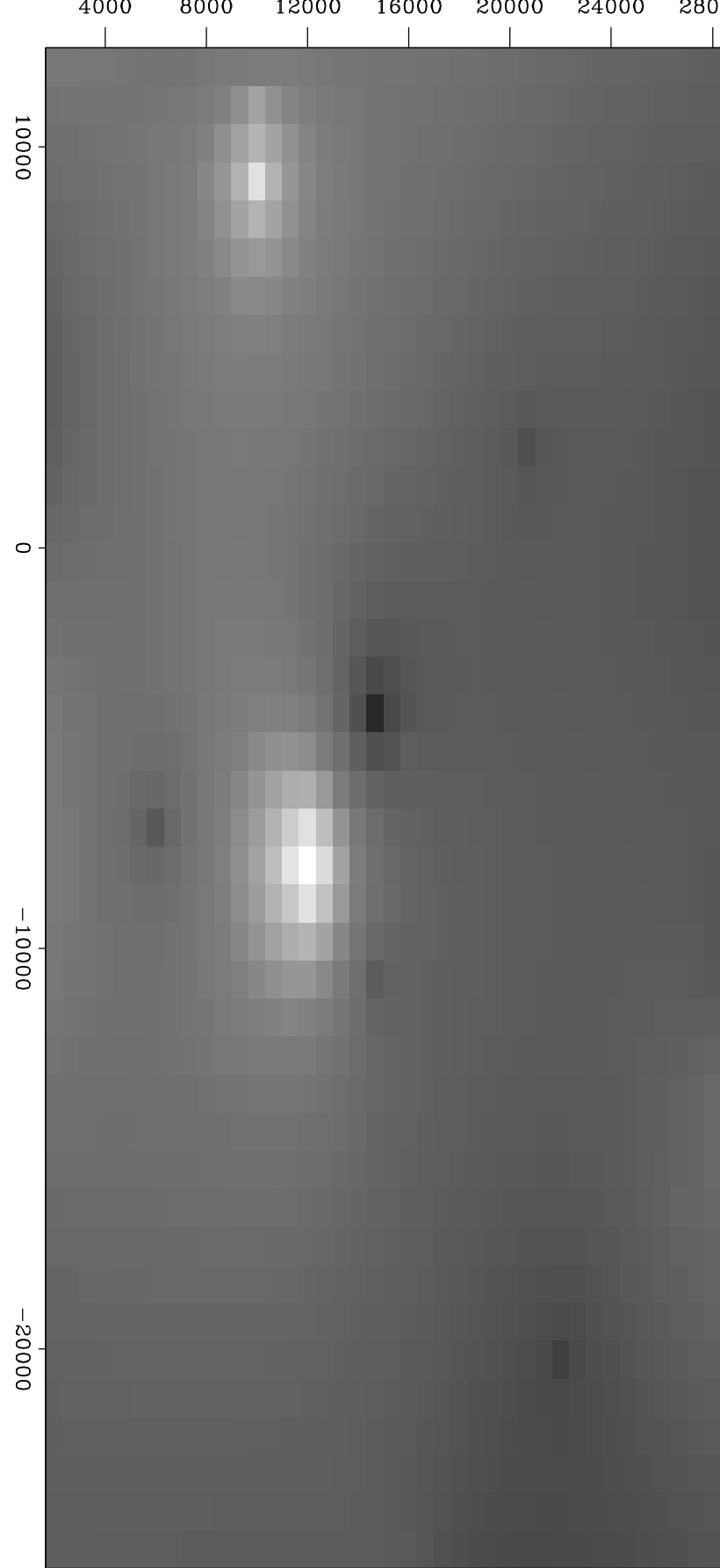
Gradient_map - Seismic
